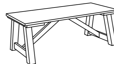
4001 Tisch mit 4-Fuss-Schräg-Streben Table avec arcs-boutants latitudinaux
